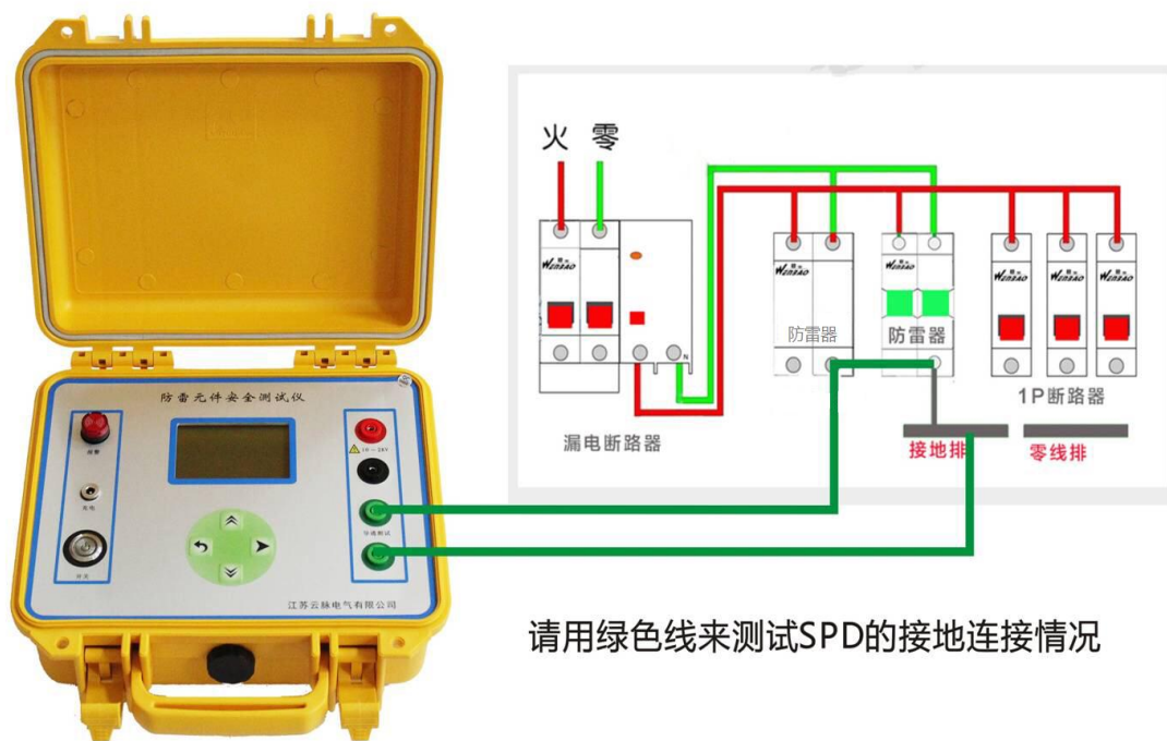
图 3 导通测试接线示意图
