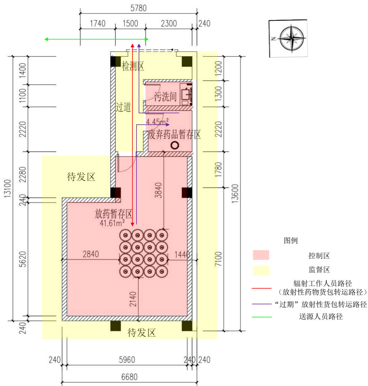
附图6 放射性药物暂存库辐射防护分区和人流物流路径规划图
