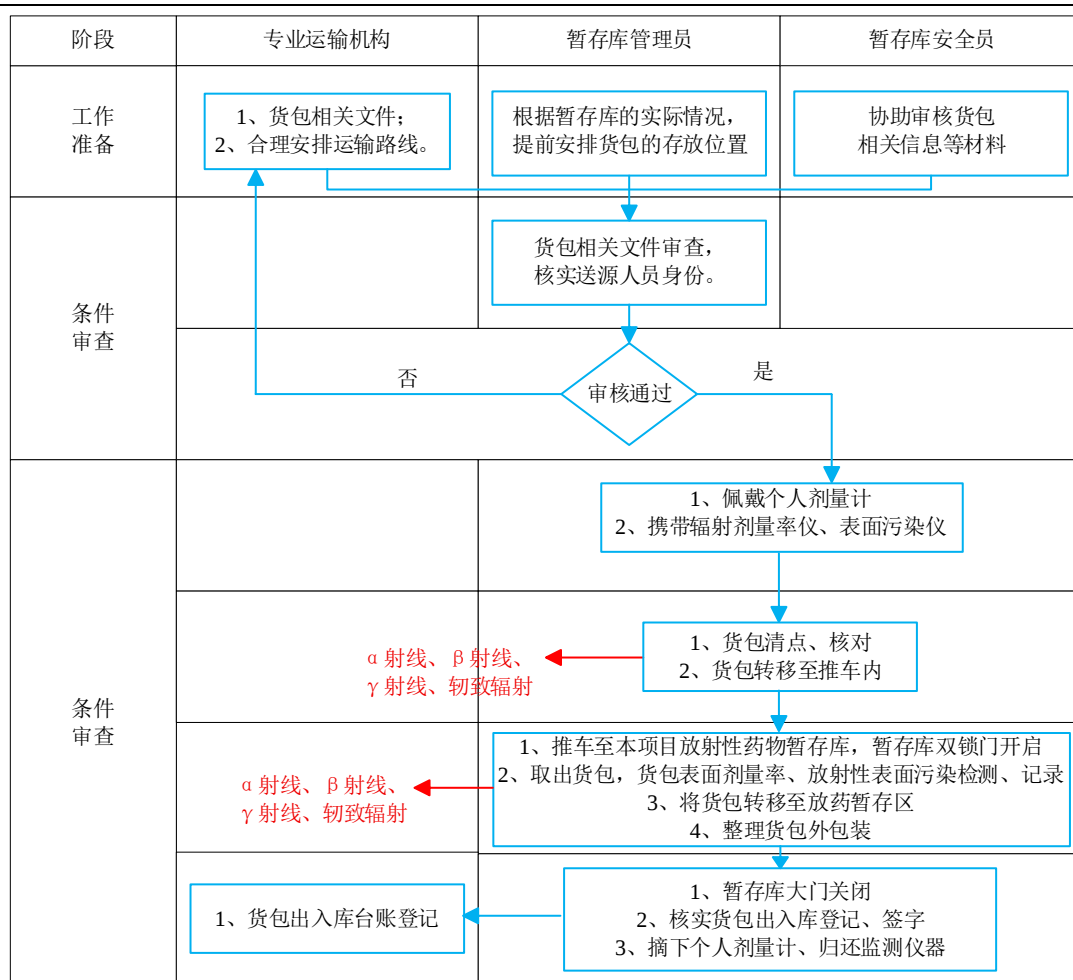
图 9-3 放射性药物货包入库工作流程及产污环节
