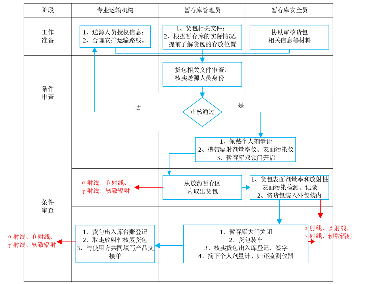
图 9-3 放射性药物货包出库工作流程及产污环节
